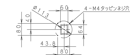
⑫ 外気取入丸合フランジ接続口詳細 (φ100)
