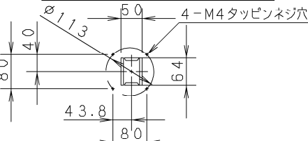
⑪ 外気取入丸合フランジ接続口詳細 (φ100)
