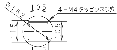
⑧ 吹出口丸合フランジ接続口詳細 (φ150)
