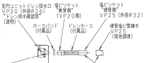
ドレンアップ立上げ寸法
