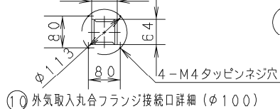
⑩ 外気取入丸合フランジ接続口詳細(φ100)
