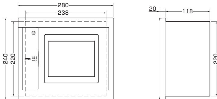
外形寸法図
