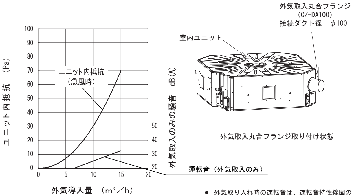
外気導入量とユニット内抵抗・運転音特性
