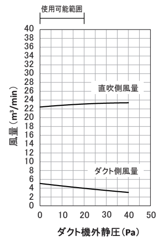
2方向吹出し
