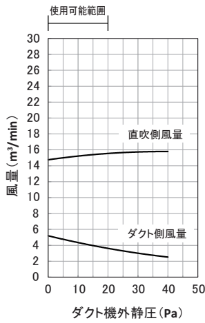
3方向吹出し
