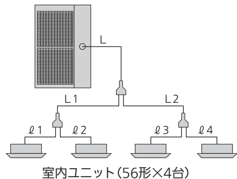
室外ユニット(224形)
