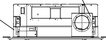
外気取入キット取付け状態
