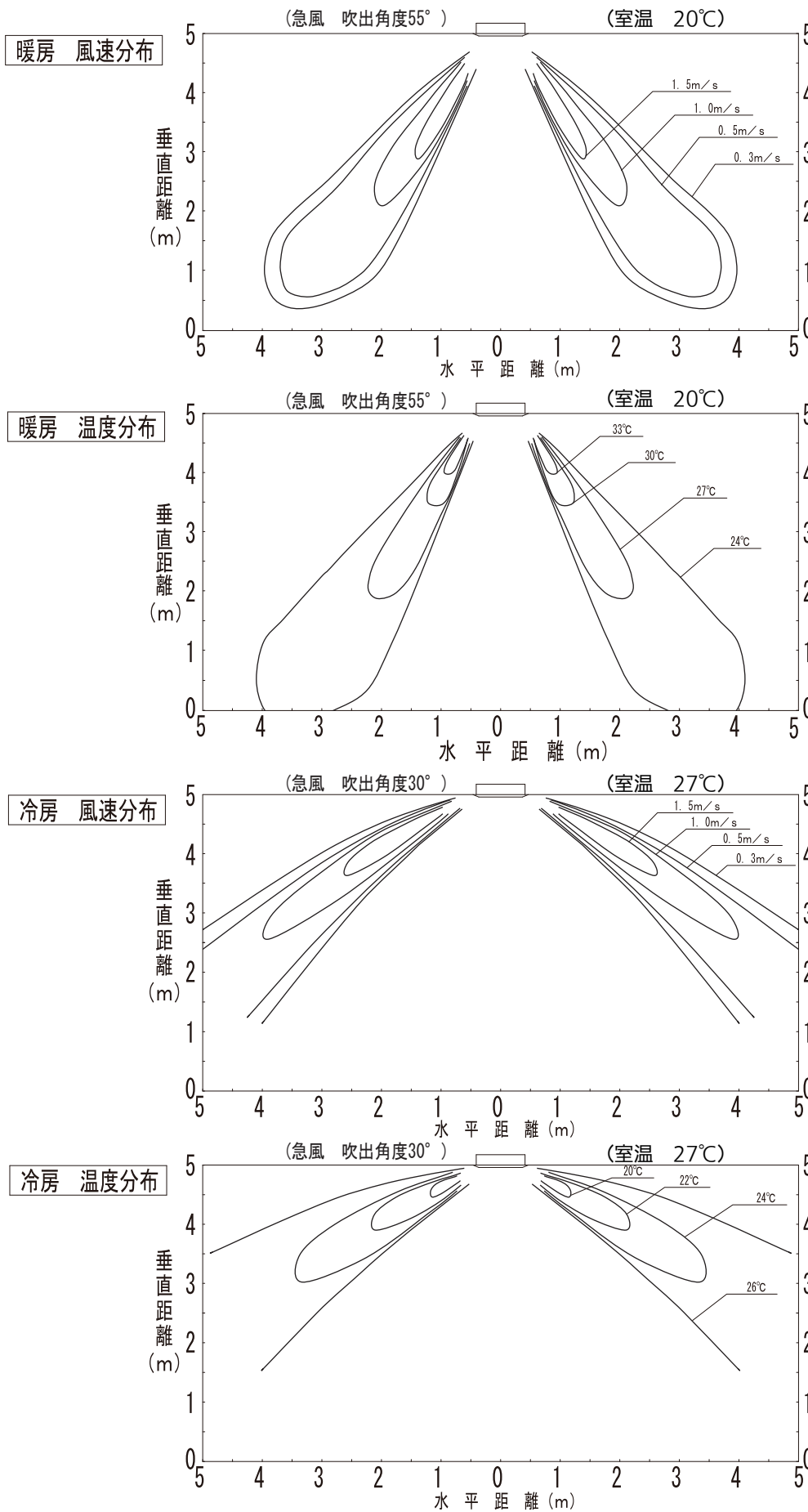
■ 4方向天井カセット形風速・温度分布（高天井仕様） 112 ~ 160形
