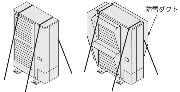
防雪ダクトを取り付けた場合
