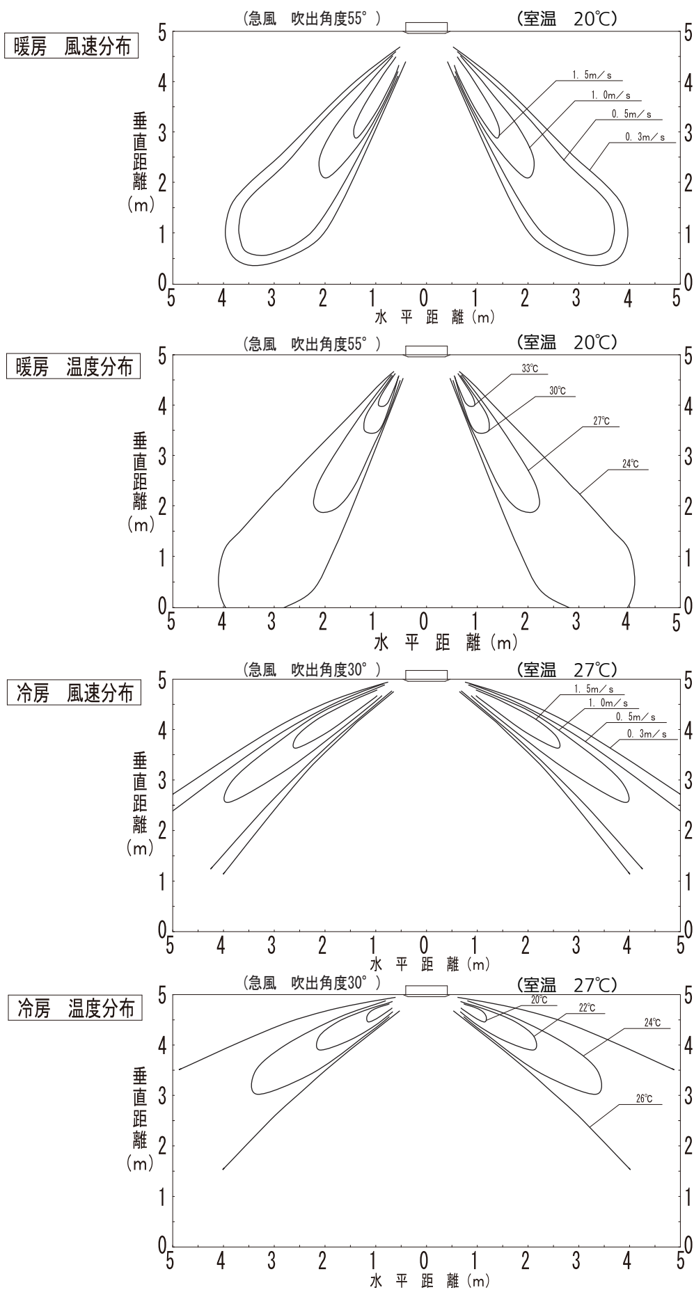
■ 4方向天井カセット形風速・温度分布（高天井仕様） 112 ~ 160形
