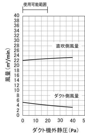
2方向吹出し
