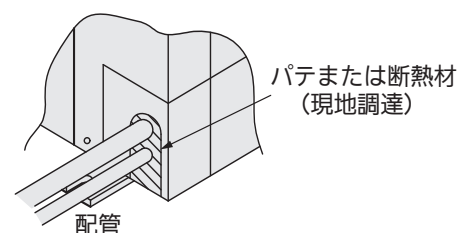
小動物侵入防止対策 図2
