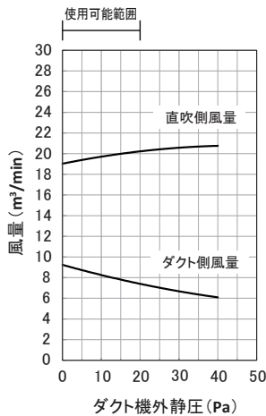
3方向吹出し
