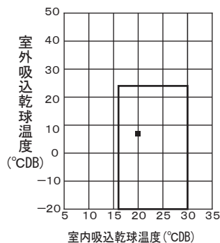
10°Cタイプ暖房時
