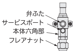
ガス管:全機種
