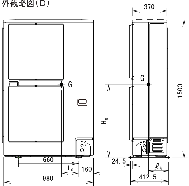
外観略図(D)
