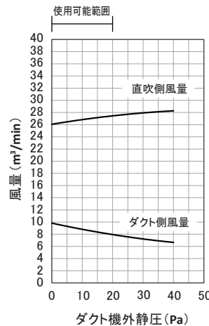
3方向吹出し
