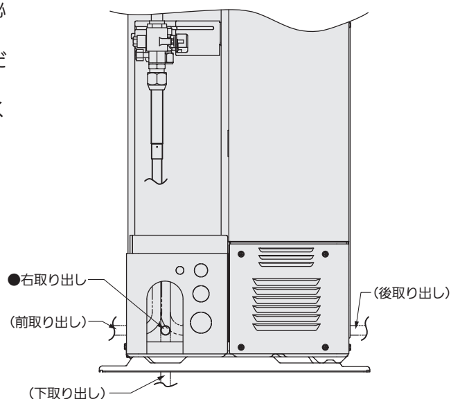
【右側面】
