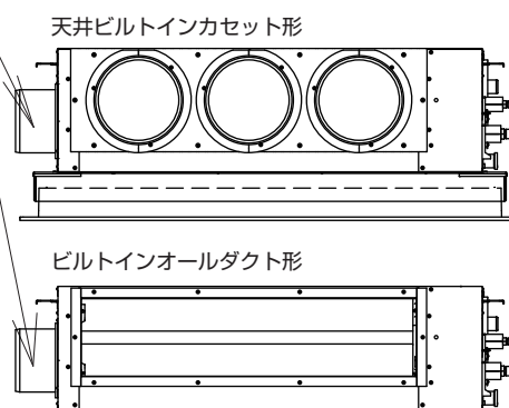
外気取入れフランジ取付け状態
