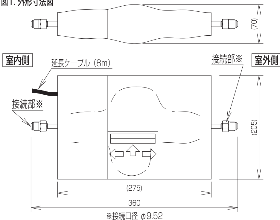
図1. 外形寸法図
