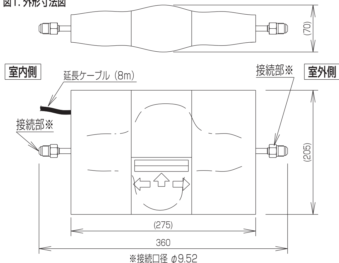
図1. 外形寸法図
