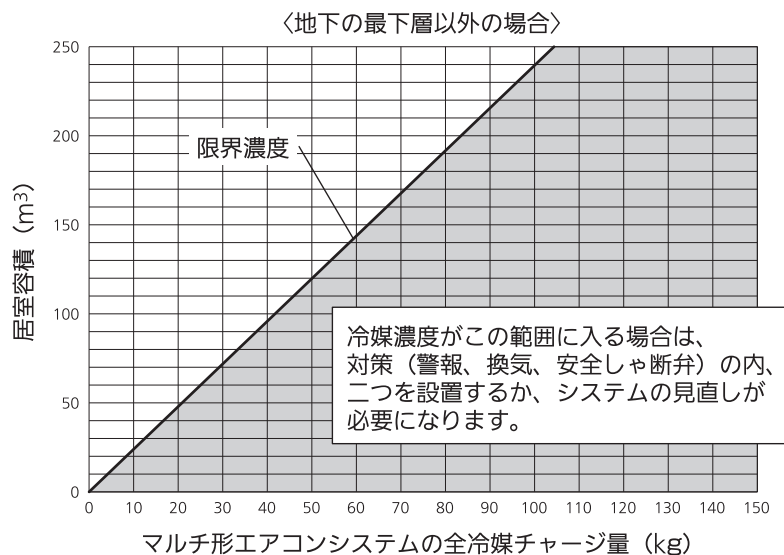
図 7：特定システムの許容冷媒チャージ量と必要な対策 [R410A 冷媒]
