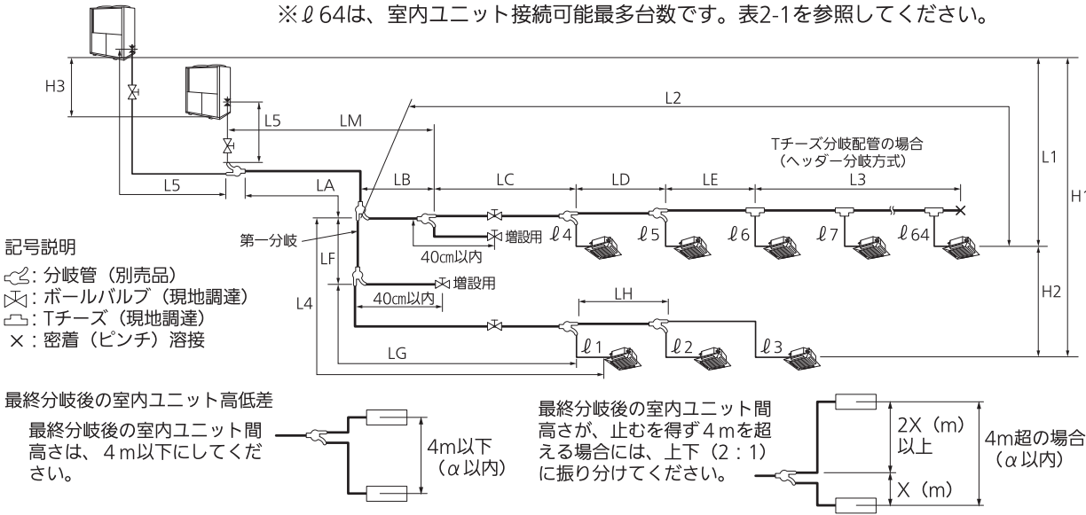
図 6：配管設計の概要
