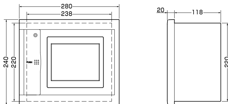
外形寸法図
