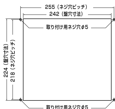
制御盤加工図
