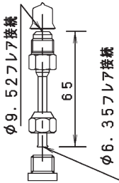
液管φ9.52用接続パイプ形状
