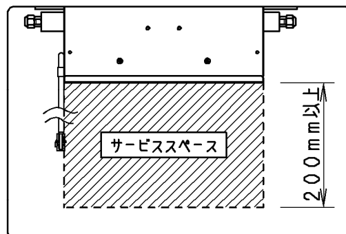
図6. サービススペースについて
