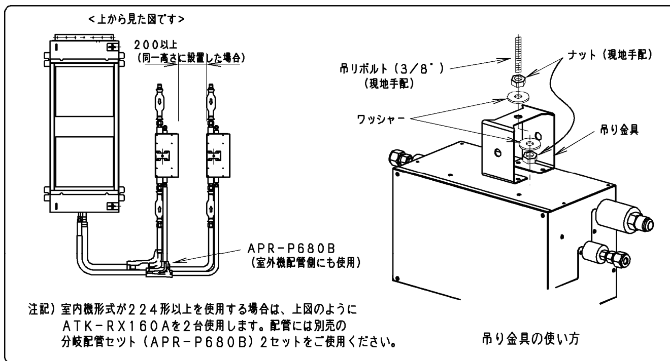
図7. ガス管弁キットの取付け例
