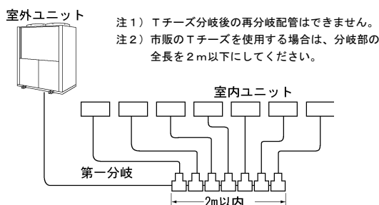
例4 ※Tチーズ分岐方式
