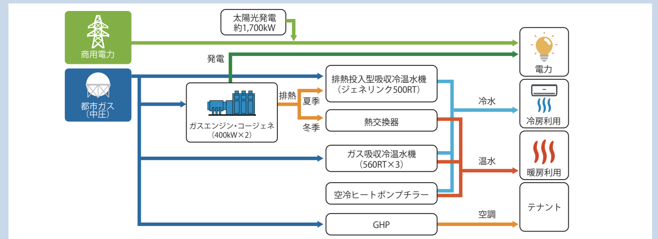
▲コージェネレーションシステム
